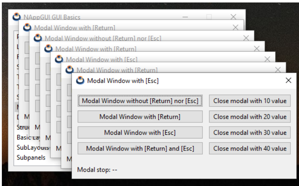
Figura 26.11: Ventanas modales.
