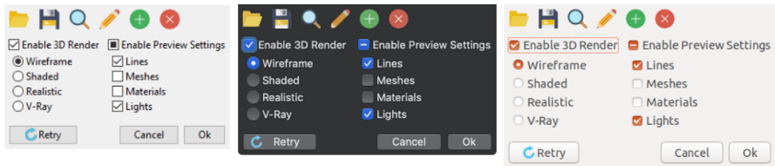
Figura 26.2: Controles Button.
