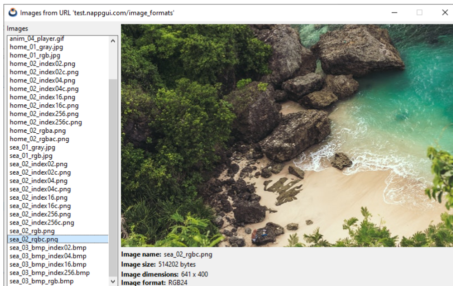
Figura 31.1: Versión Windows
