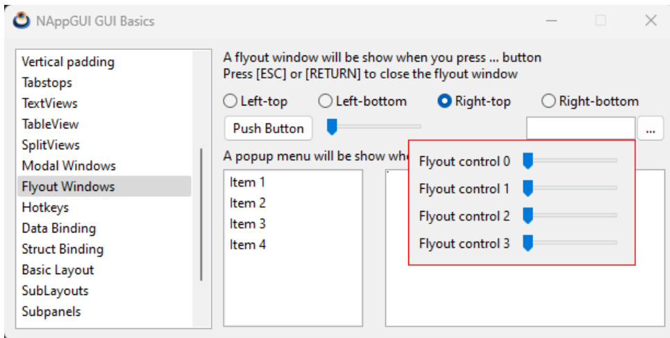
Figura 26.12: Ventanas superpuestas.
