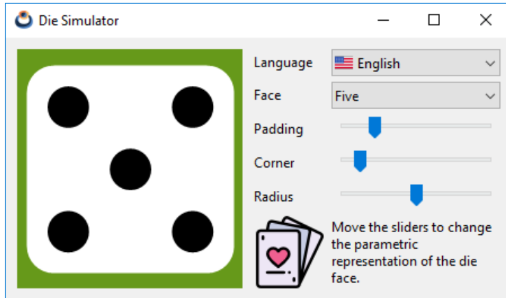
Figura 9.1: Aplicación Die .
