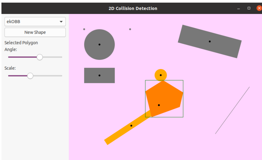
Figura 28.3: Versión Linux.
