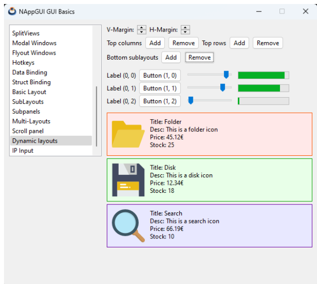
Listado 26.18: demo/guihello/dynlay.c
