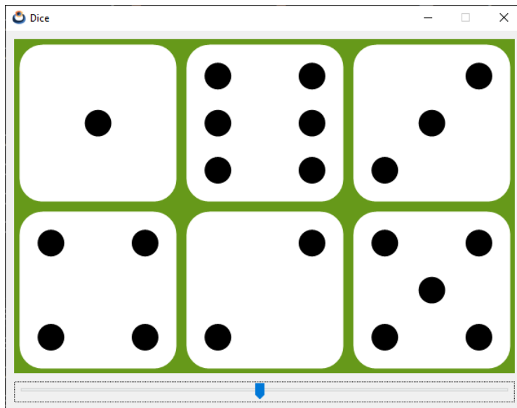
Figura 9.2: Aplicación Dice .
