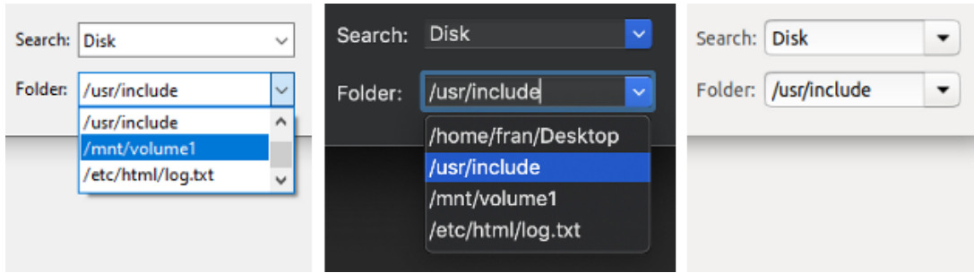
Figura 26.4: Controles Combo.
