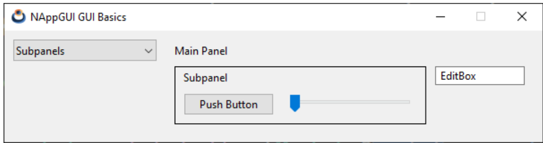
Figura 26.16: Subpaneles.
