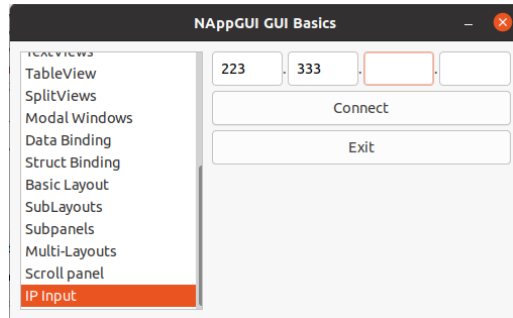
Listado 26.19: demo/guihello/ipinput.c
