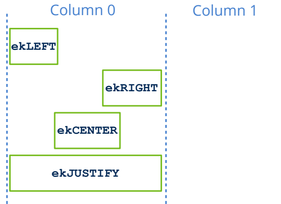
Figura 18.62: Alineación horizontal.
