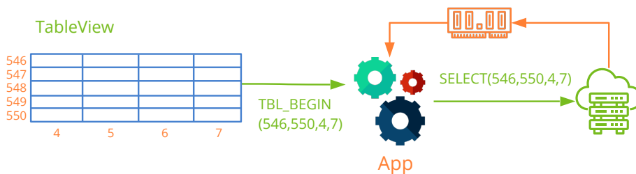
Figura 18.44: Uso de caché de datos.
