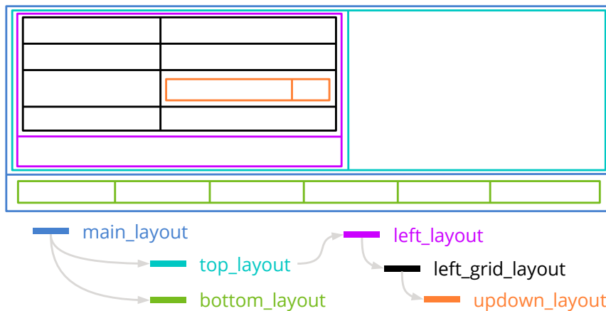
Figura 18.57: Sublayouts necesarios para componer el panel de (Figura 18.56).
