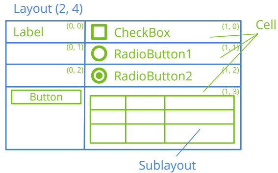
Figura 18.60: Celdas en el interior de un Layout
