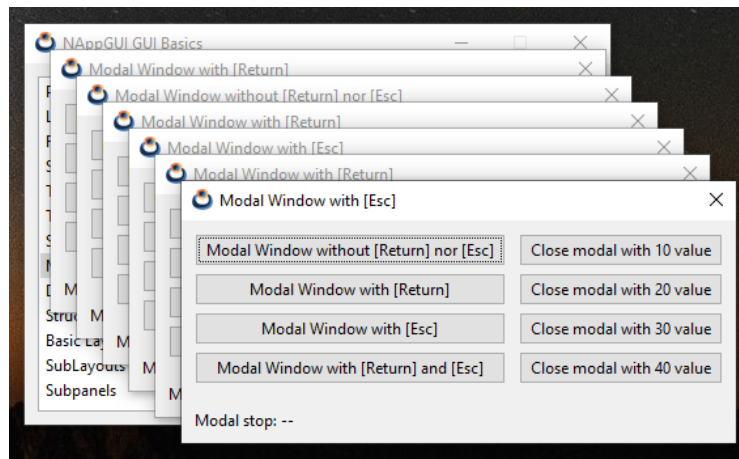
Figura 18.75: Varias ventanas modales.
