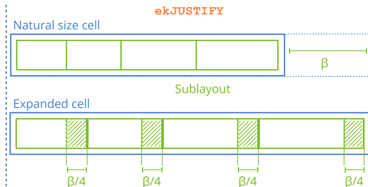
Figura 18.58: Cuando el tamaño del sublayout viene dado por condiciones externas, se reparte por igual el exceso de píxeles entre las columnas (expansión horizontal) y filas (expansión vertical).
