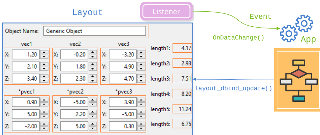
Figura 18.79: Notificación de cambio de valor al programa principal.
