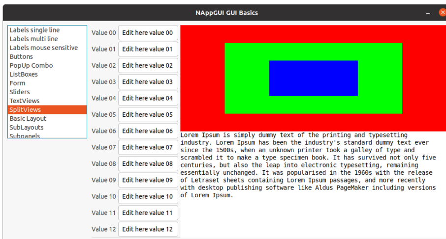
Figura 18.51: SplitView en Linux.
