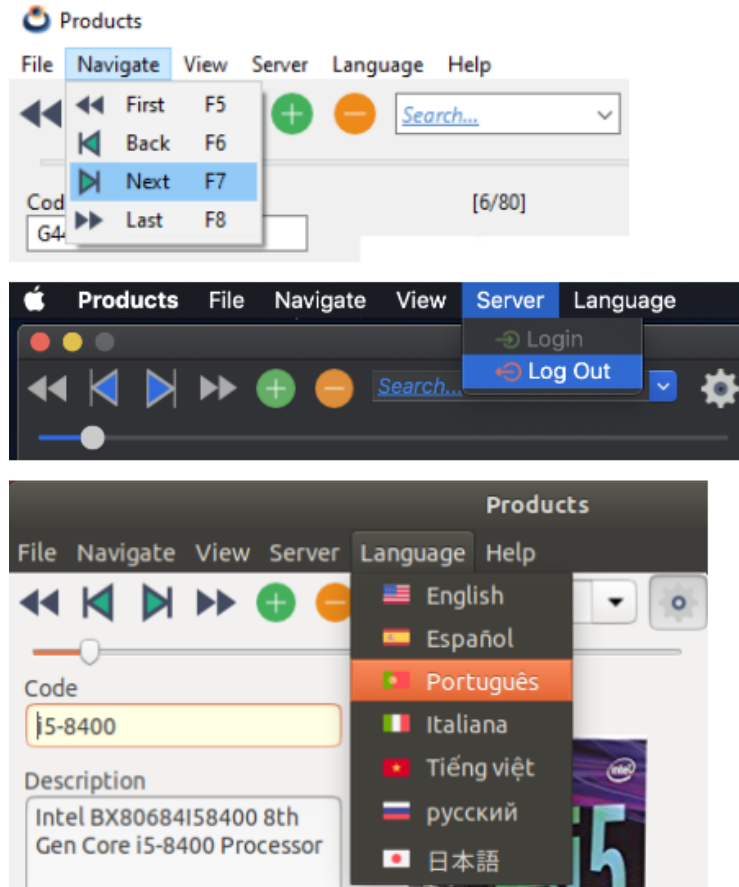
Figura 18.80: Barra de menú en Windows, macOS y Linux.
