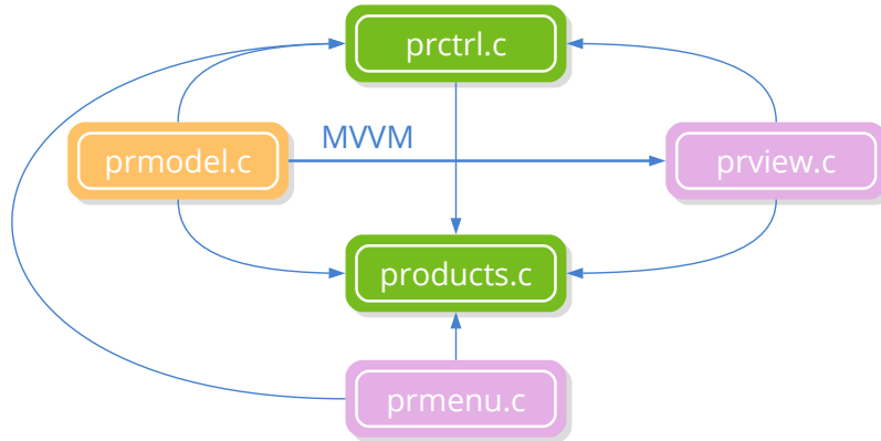
Figura 25.4: Módulos MVC que componen la aplicación.
