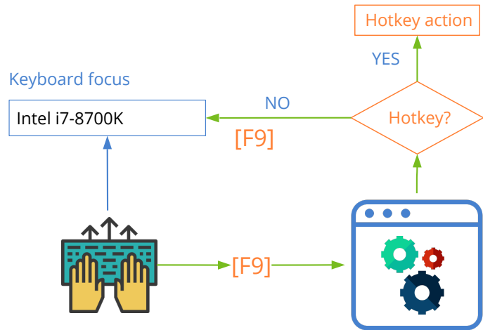
Figura 18.76: Procesamiento de un atajo de teclado.
