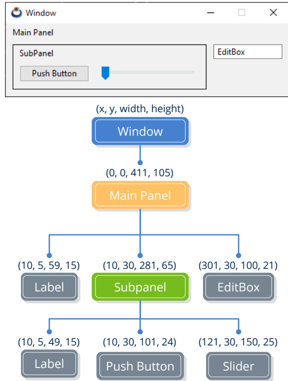
Figura 18.62: Jerarquía de ventana.
