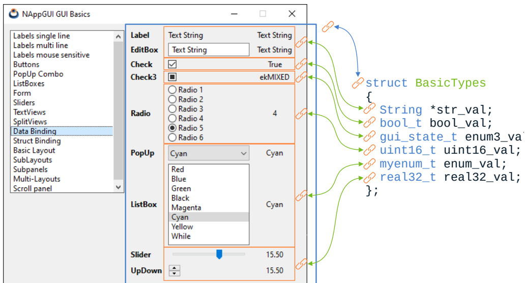
Figura 18.77: Sincronización automática de datos con la interfaz de usuario.
