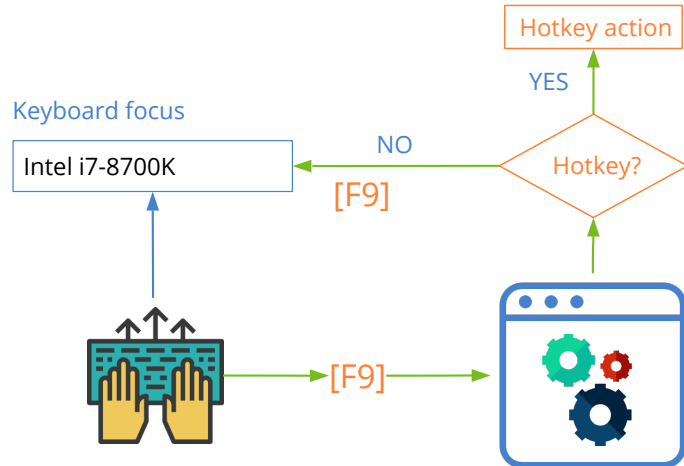
Figura 18.75: Procesamiento de un atajo de teclado.
