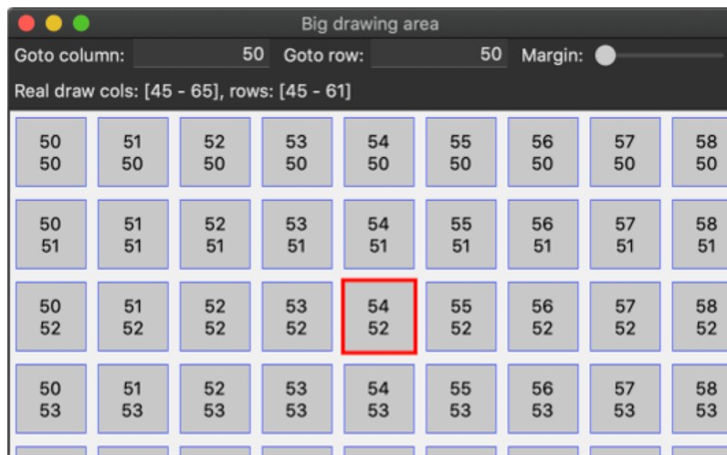
Figura 30.2: Versión macOS.
