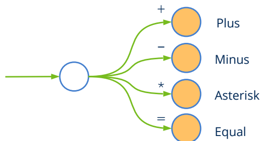
Figura 15.19: Autómata finito que reconoce algunos símbolos.
