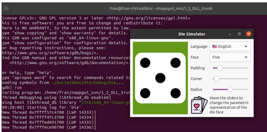
Figura 8.15: Depurando Die con GDB desde el terminal.
