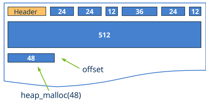
Figura 15.2: Reserva de un nuevo bloque de memoria con heap_malloc() .
